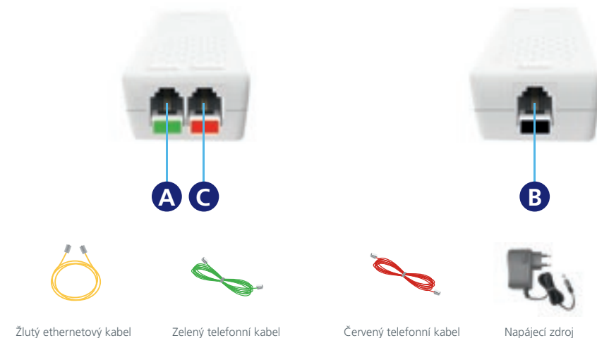
Rozbočovač PHONE, MODEM
